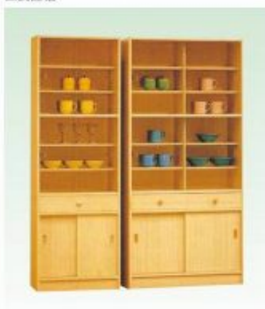
食器棚 小: W550×D300×H1200mm 中: W600×D300×H1600mm 大: W650×D300×H1600mm
